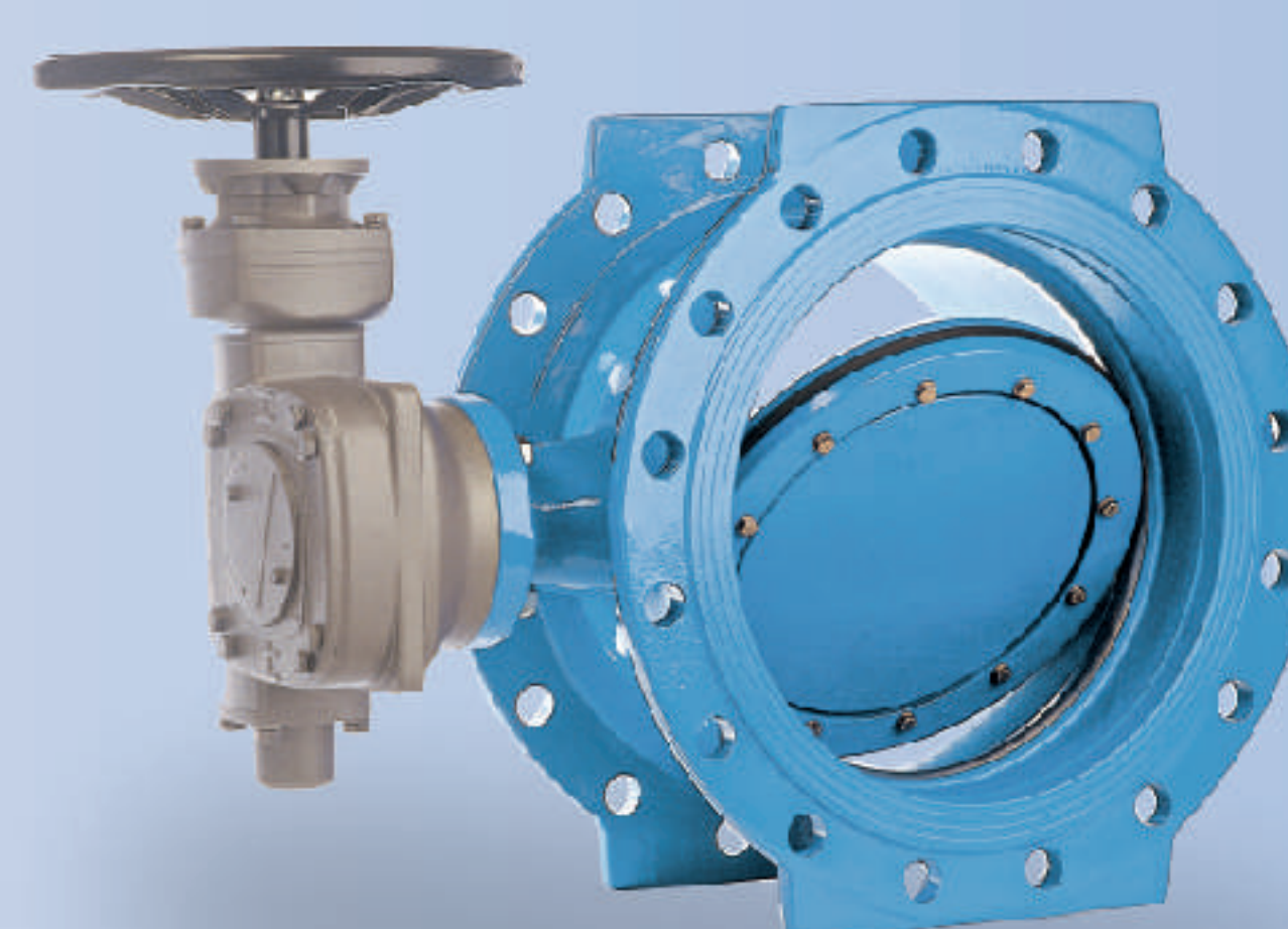
Tipo Brida De Doble Excentricidad: DN 150 a 2.000mm (PN 10, 16 y 25 Bar)
